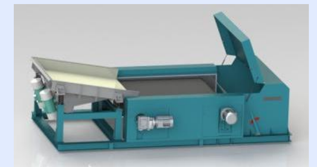
Magnetabscheider nach dem Foucault-Strom-Prinzip (patentiert)
