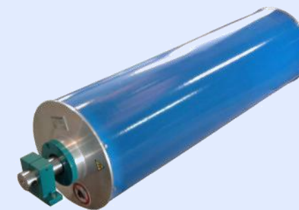
Trommeln mit hoher magnetischer Intensität mit rotierender Hülle aus Verbundmaterial und mit Polyurethanbeschichtung
